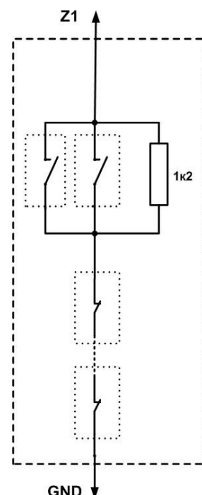
Рисунок 11 Подключение извещателей пожарного шлейфа
