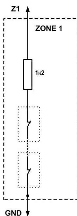
Рисунок 11 Подключение извещателей пожарного шлейфа
